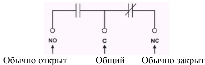
Рисунок 6 – Показ соединений реле в несрабатанном состоянии
